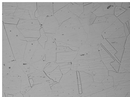
健全な組織(SUS304)
