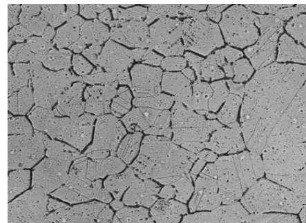
鋭敏化した組織(SUS304)
