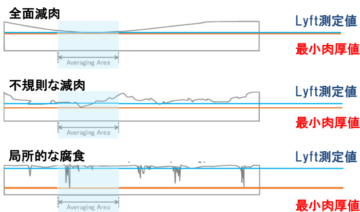
各種減肉形態におけるLyft測定値
