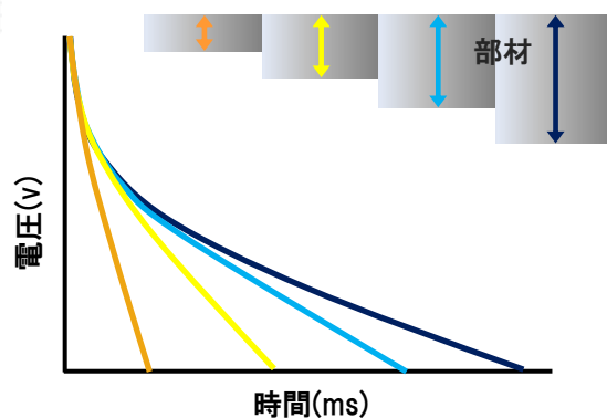
各板厚における減衰率変化
